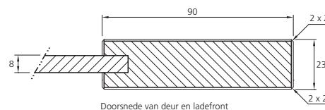
Doorsnede van deur en ladefront
