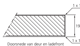
Doorsnede van deur en ladefront
