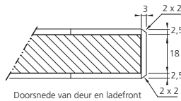
Doorsnede van deur en ladefront
